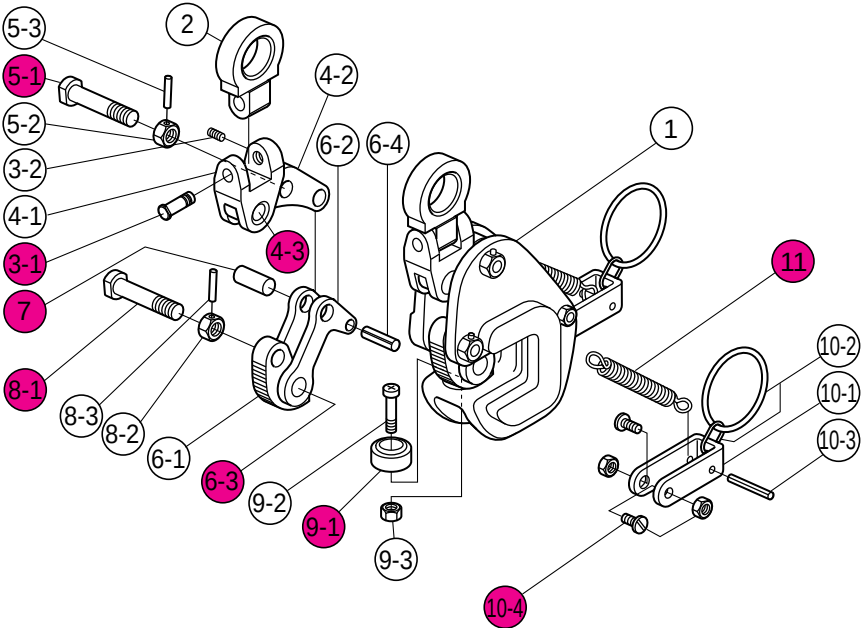
分解構造図
