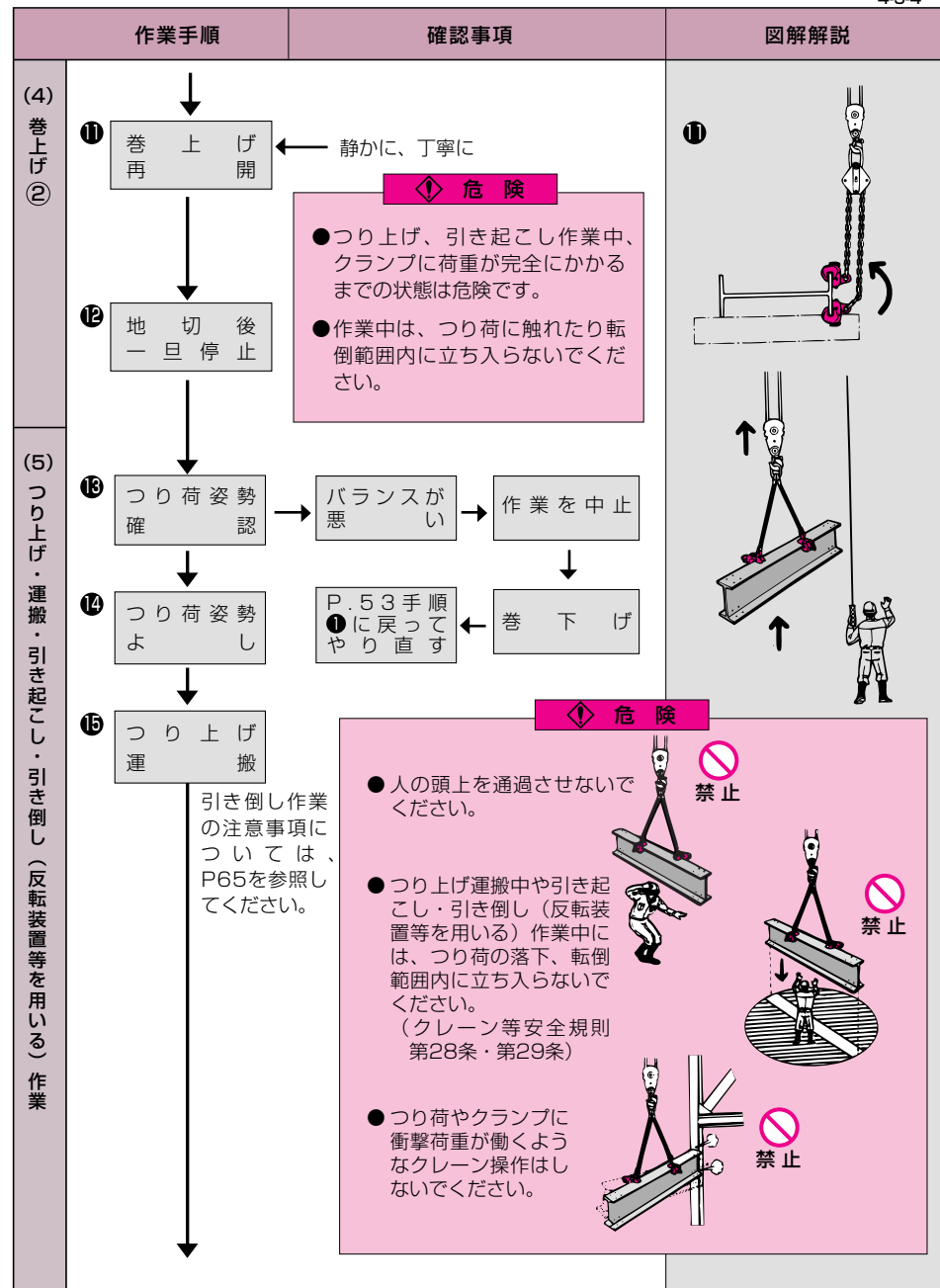
横つり用クランプ
